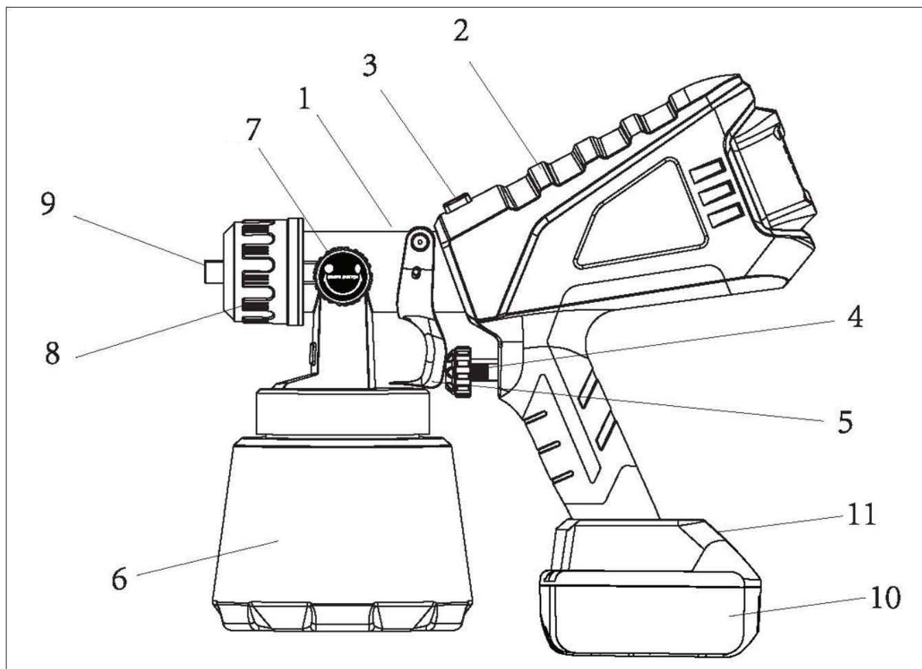
Рис. 1. Общий вид
