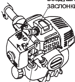
Ручка стартера
